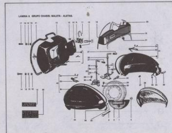
GRUPO CHASIS
