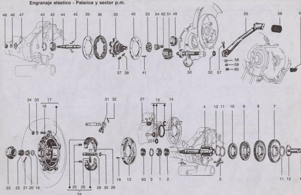
LAMINA 3 GRUPO MOTOR: Engranajes cambio-tambor - Zapatas traseras - Engranaje elástico - Palanca y sector p.m.
