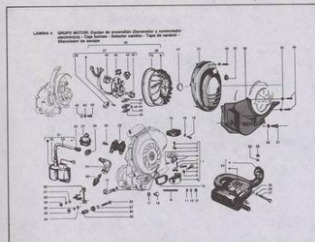
GRUPO MOTOR
