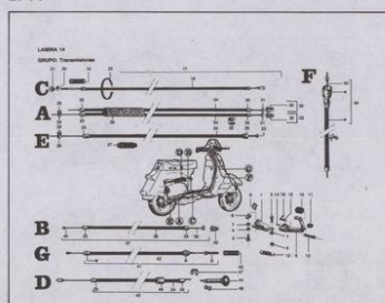
GRUPO TRANSMISIONES
