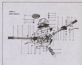
GRUPO MANILLAR
