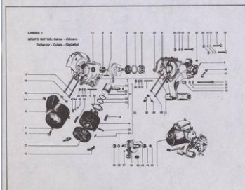
GRUPO MOTOR
