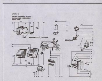
GRUPO ELECTRICO
