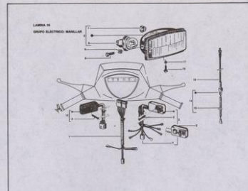
GRUPO ELECTRICO
