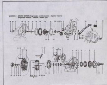
GRUPO MOTOR
