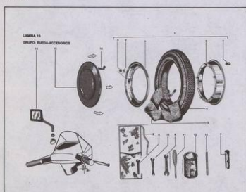
GRUPO ACCESORIOS
