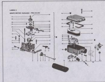
GRUPO MOTOR
