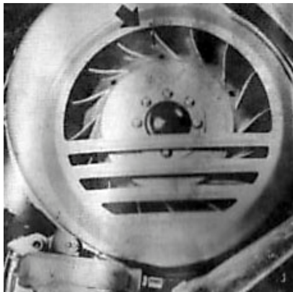
Fig. 42 Marcas de referencia en el rotor y tapa de caracol.
