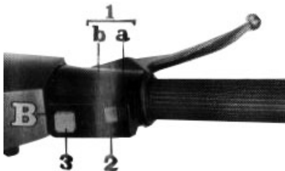
Fig. 16 bis Conmutador de luces con pulsador de arranque.
