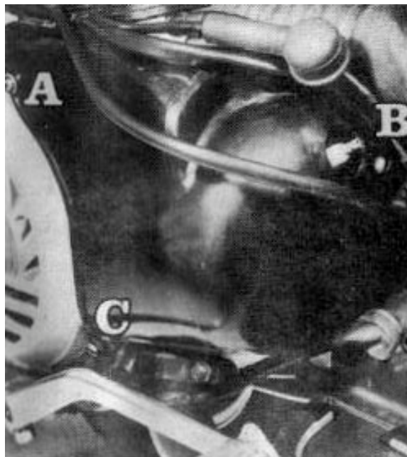
Fig. 26 Desmontaje deflector de refrigeración.
