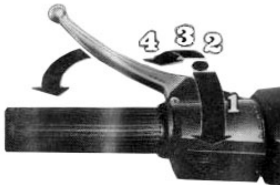
Fig. 21 bis Cambio de velocidades. Mando cambio combinado con palanca embrague.
