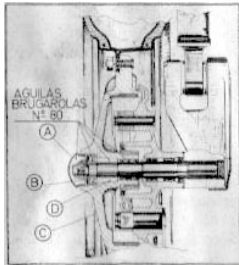
Fig. 44 bis Engrase tambor freno delantero.
