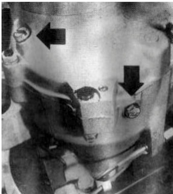
Fig. 25 Orificios de llenado y vaciado del aceite.
