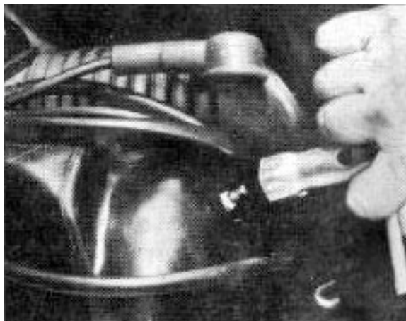
Fig. 24 Desmontaje bujía.
