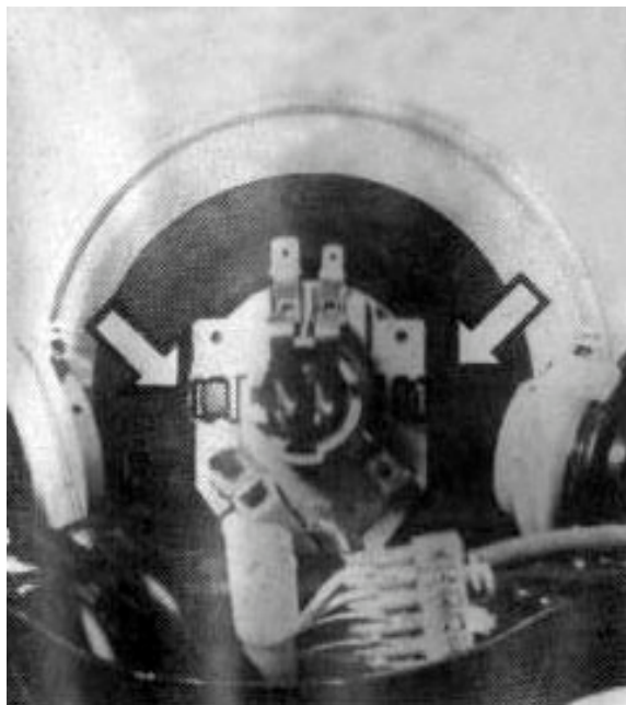
Fig. 36 Acceso lámpara del faro.
