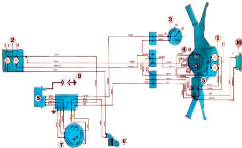
Fig. 18 Esquema eléctrico Vespa PX 150 E.
