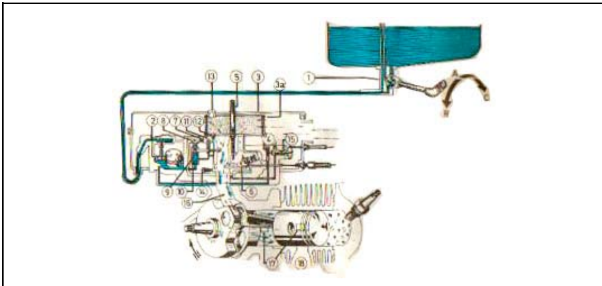
Fig 22 Esquema de alimentación y distribución
