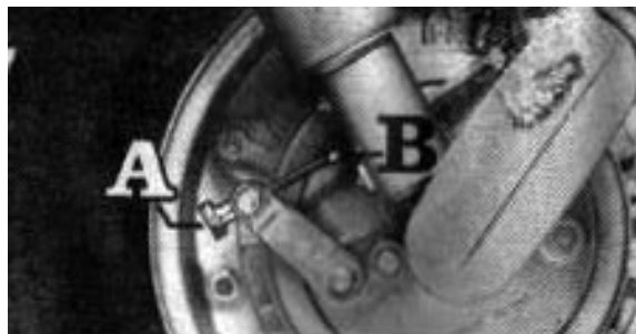
Fig. 33 Regulación freno delantero.
