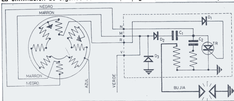
Fig. 19 E.—VESPA PK 125 · 75 S. Solución FEMSA
