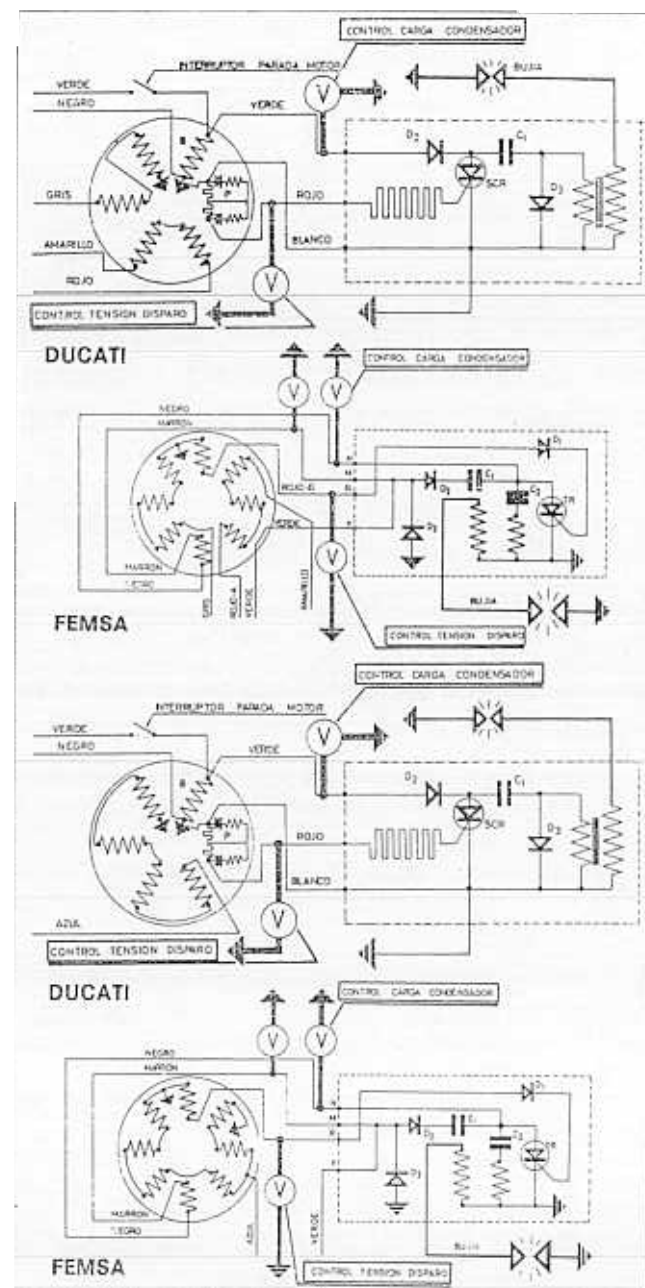
Fig. 23 E.—Control de tensión de carga del condensador y tensión de disparo
