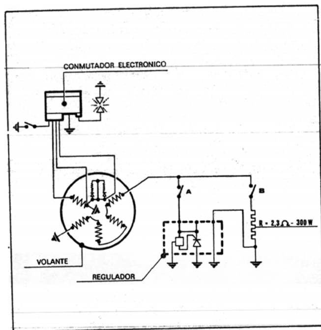
Fig. 29 E.—Control circuito B. T.
