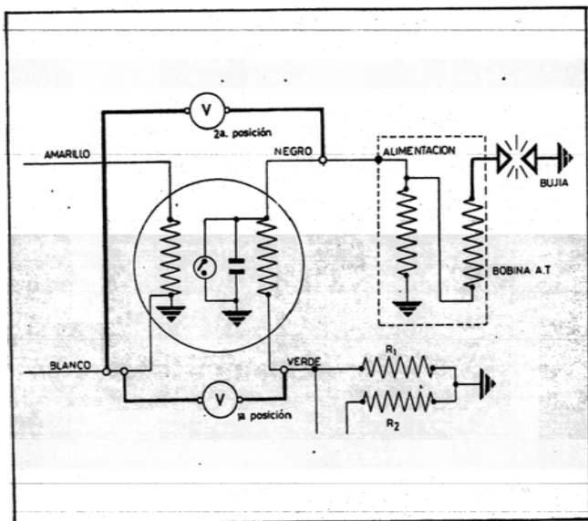
Fig. 4 E.—Control circuito de encendido
