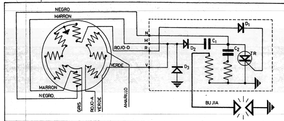
Fig. 20 E.—VESPA PK 125 · 75 S ELESTART. Solución FEMSA
