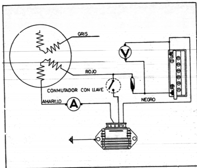
Fig. 26 E.—Control regulador circuito c. c.
