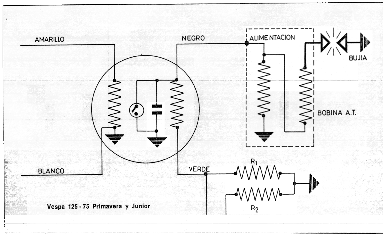
Fig. 3 E.—Esquema eléctrico. Grupo de encendido
