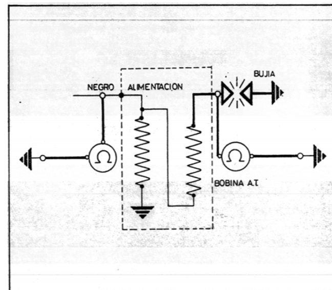
Fig. 6 E.—Control bobina de A. T.
