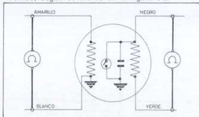
Fig. 8 E.—Control estático del estátor
