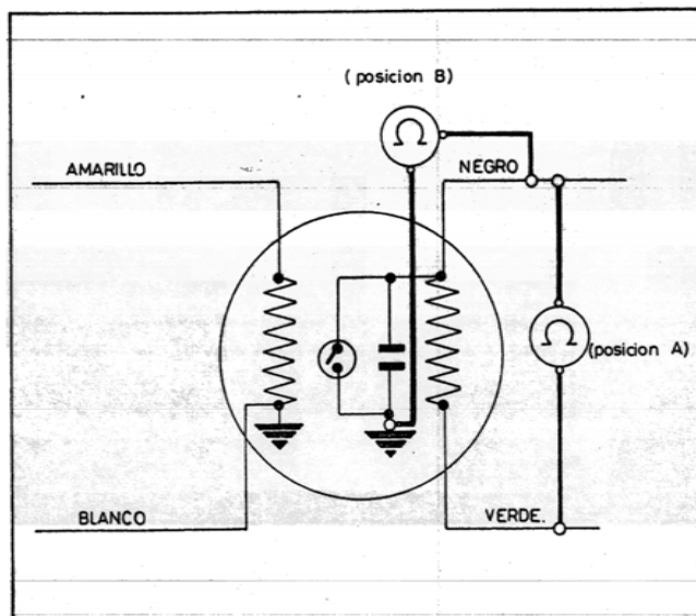
Fig. 5 E.—Control volante magnético
