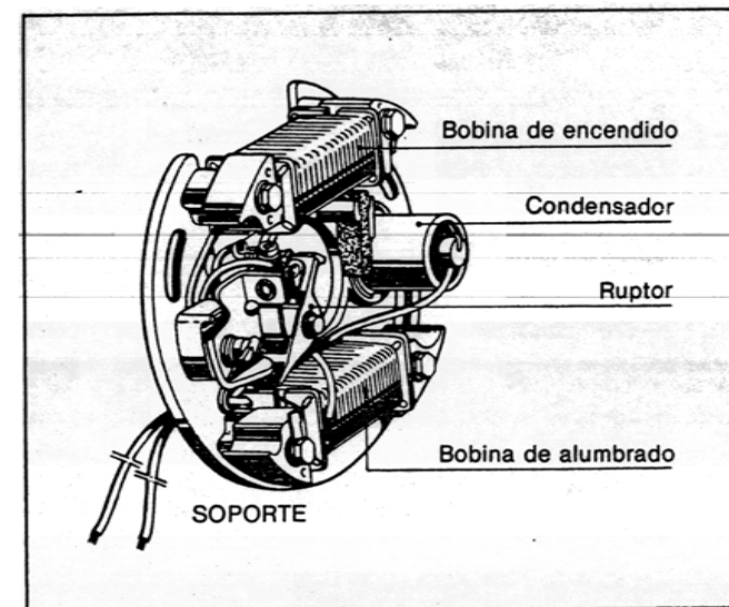
Fig. 1 E.—Estátor (soporte bobinas)
