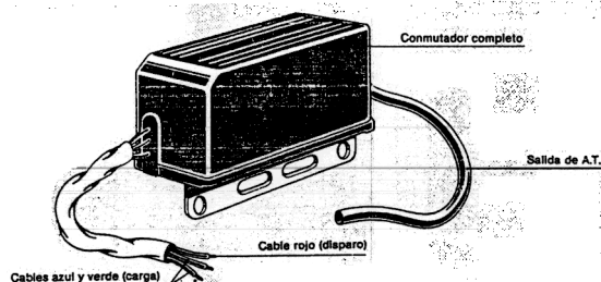
Fig. 17 E.—Conmutador electrónico, solución FEMSA
