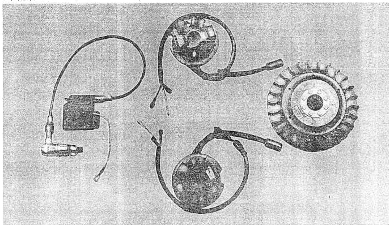
Fig. 18 E.—Componentes del equipo de encendido, solución DUCATI
