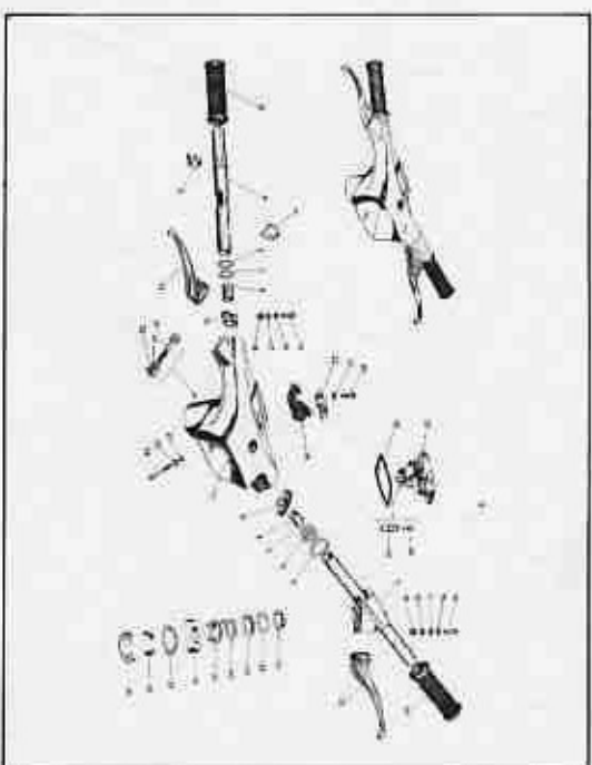
GRUPO DIRECCION - MANILLAR
