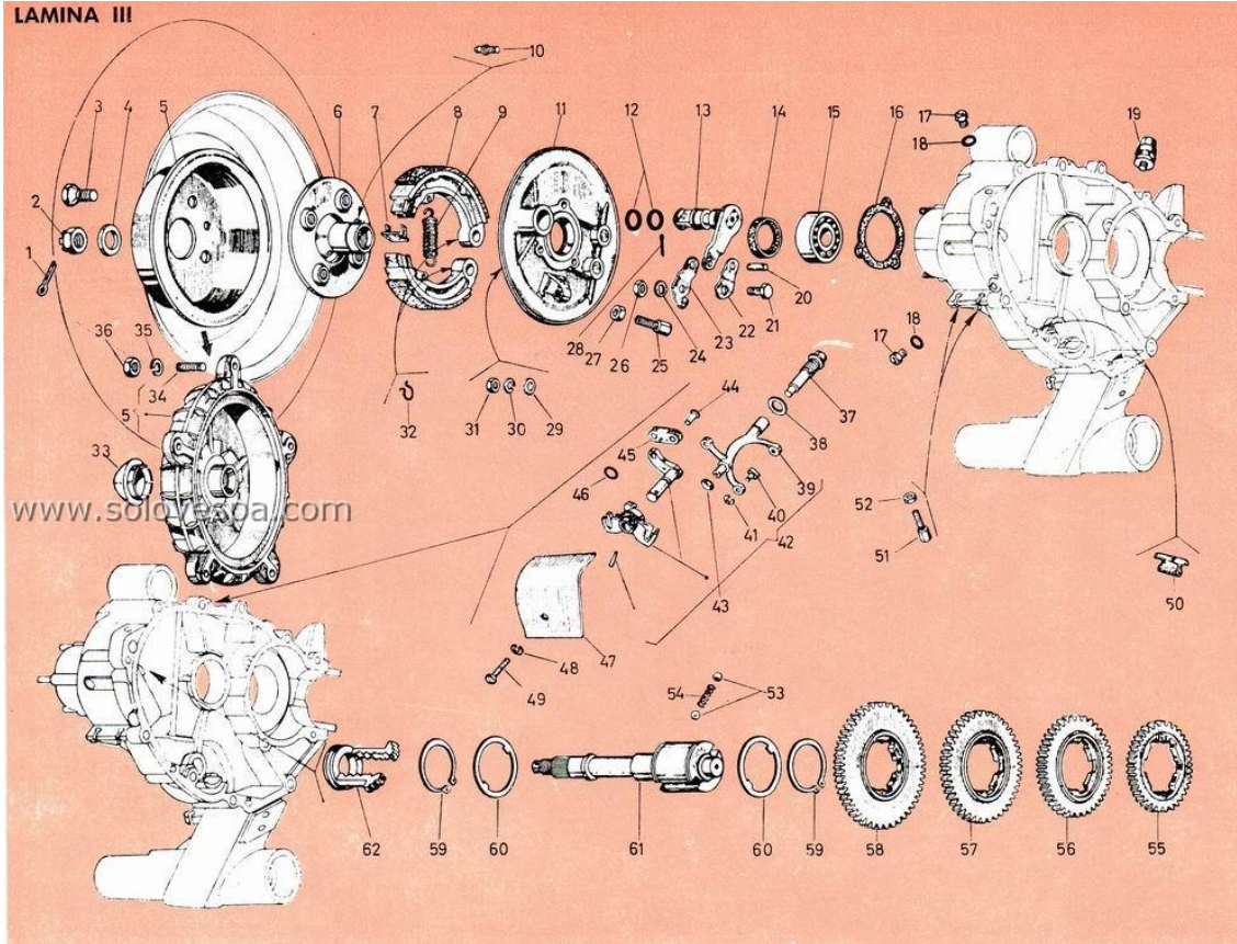
GRUPO MOTOR: Tambor freno trasero - Engranajes cambio
