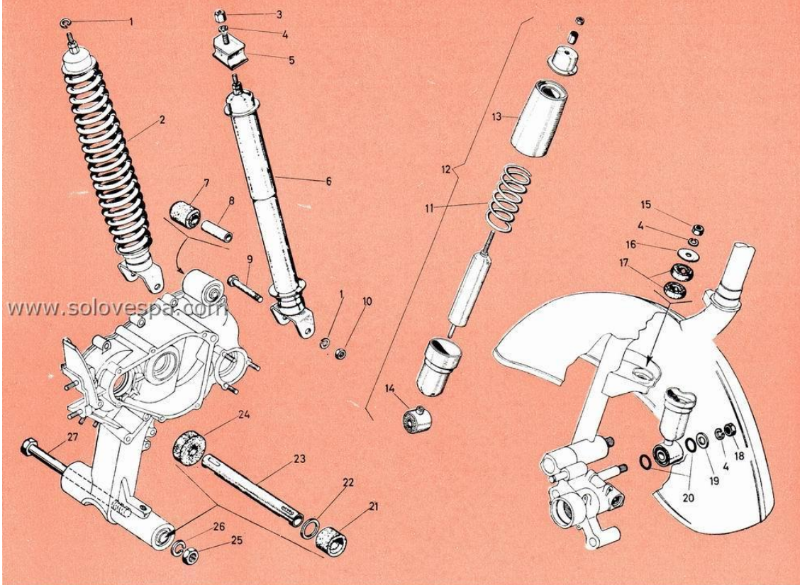
GRUPO SUSPENSIONES: Amortiguador delantero y trasero
