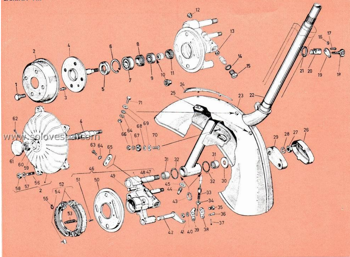
GRUPO DIRECCION - MANILLAR: Dirección - Cubo y eje rueda - Tambor freno - Dispositivo antihurto
