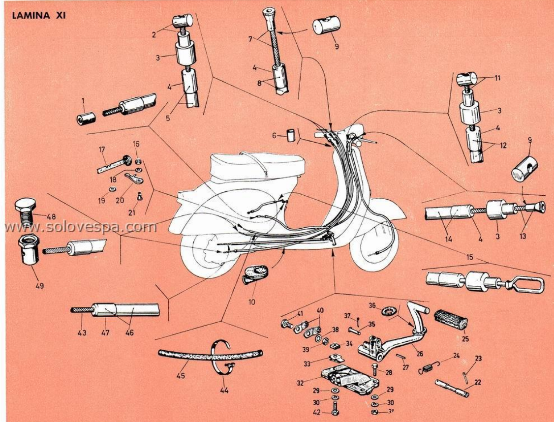
GRUPO TRANSMISIONES: Transmisiones - Pedal freno trasero
