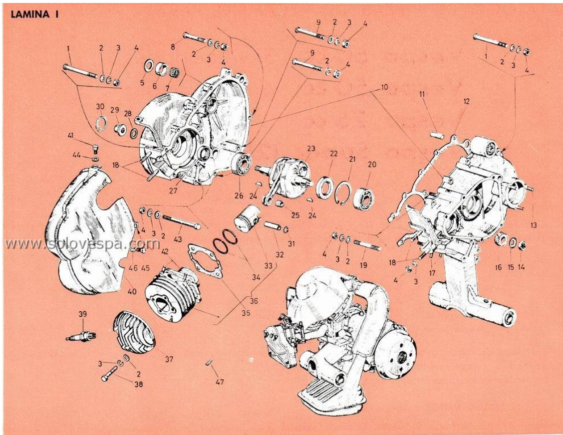
GRUPO MOTOR: Carter - Cilindro - Cigüeñal
