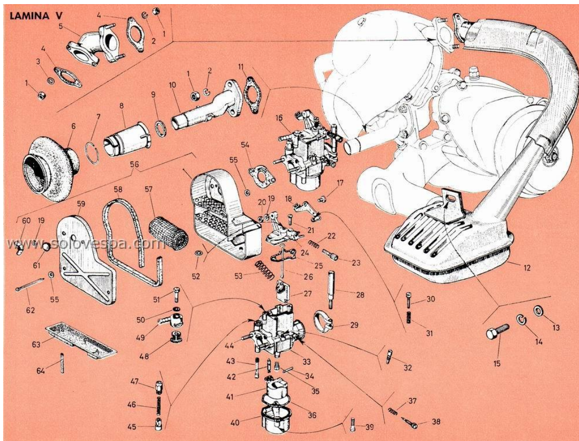
GRUPO MOTOR: Carburador - Filtro de aire
