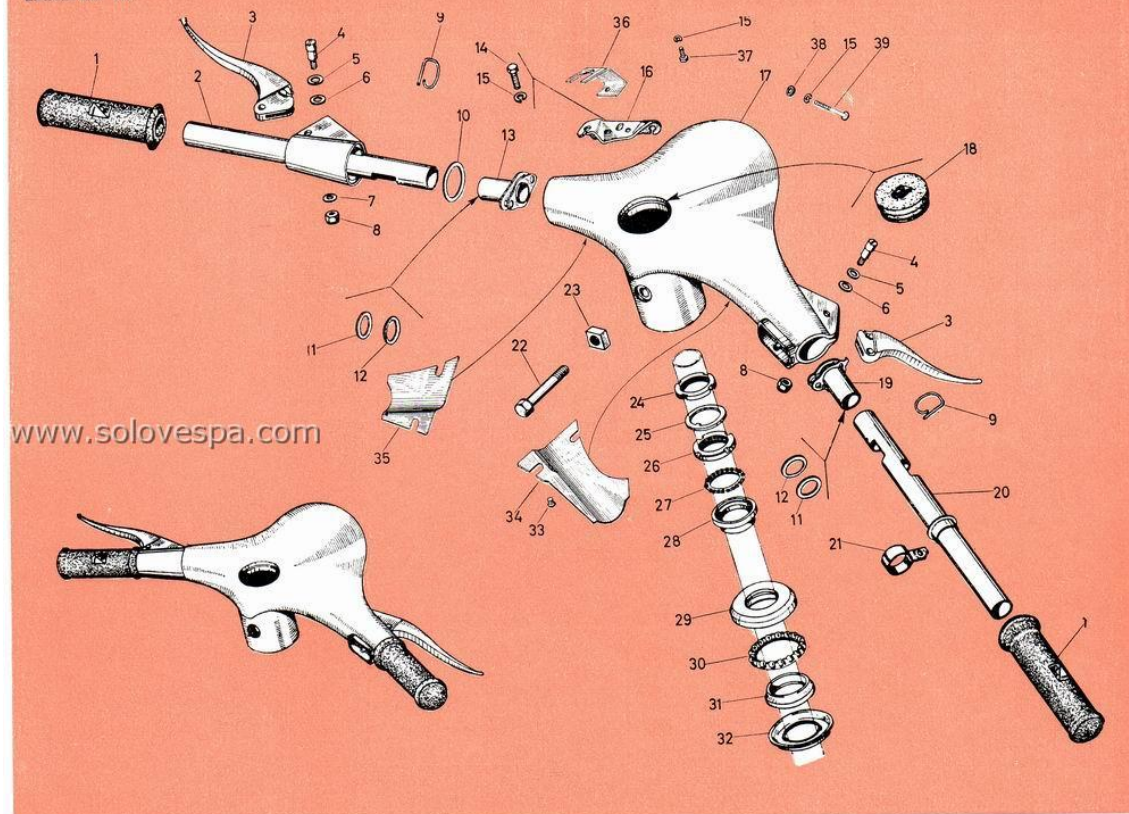
GRUPO DIRECCION-MANILLAR: Manillar - Cojinetes dirección
