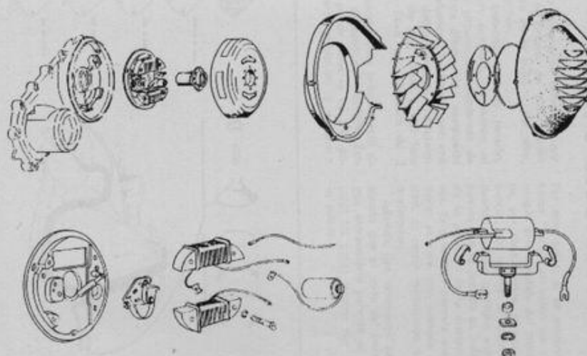
GENERADOR DE CORRIENTE Y TURBINA DE REFRIGERACION
