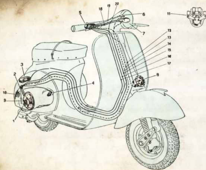
Fig. 8 — Instalación eléctrica.
