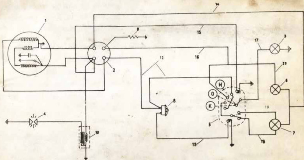
Fig. 8 bis. — Esquema de la instalación eléctrica.
